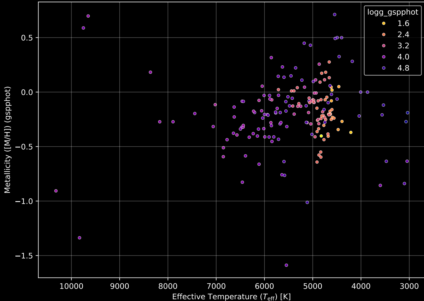
APOGEE DR17 Field: [CVZTILE_103+33_btx] Stellar Population Parameters (n= 178)
